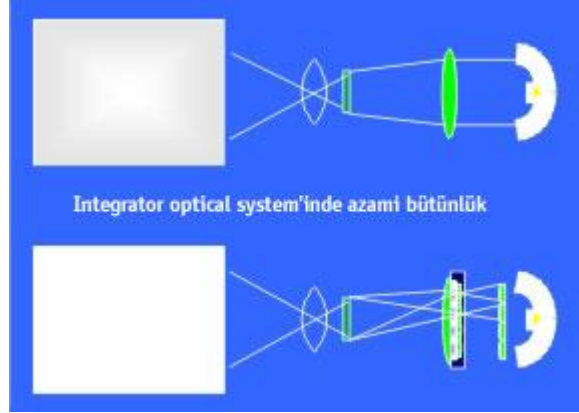
Şekil 3.6: Polarize dönüşüm şeması
