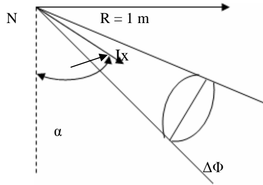
Şekil 1.5: Işık şiddeti
