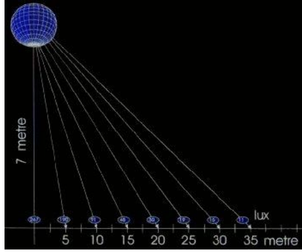
Şekil 2.6: 7 metrelik balon ışık
