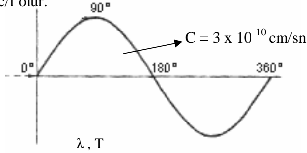
Şekil 1.2: Dalga boyu
