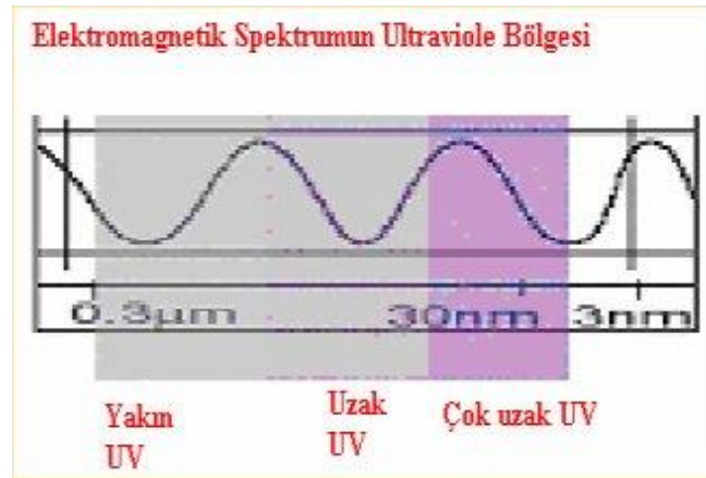
Şekil 3.2: Işık spektrumu
