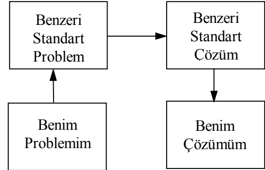
Şekil 1. Genel Problem Çözme Modeli
